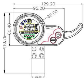
Вид спереди
